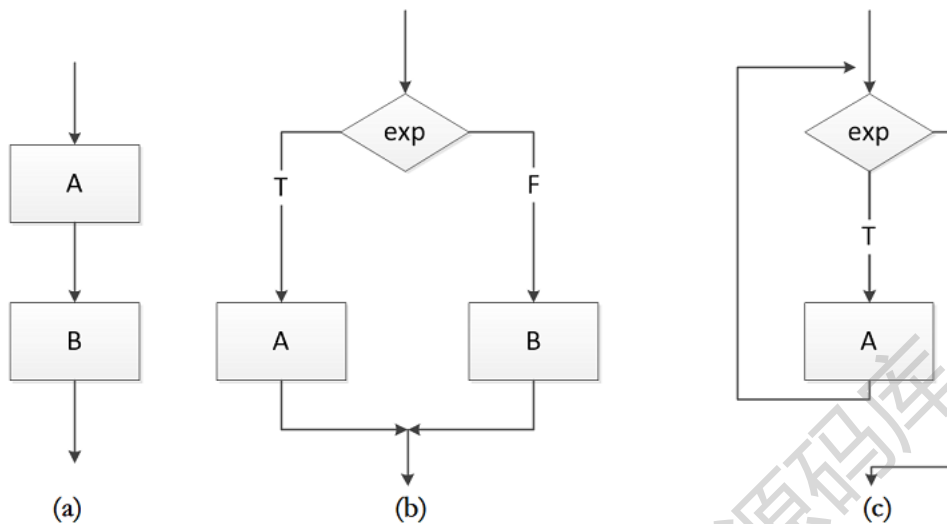
(a)顺序结构，先执行A再执行B；(b)IF-THEN-ELSE 型选择(分支)结构； (c)DO-WHILE 型循环结构
